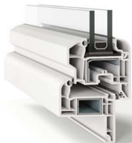
Anta semicomplanare SOFTLINE 70 AD abbinata a telaio SWINGLINE 70 AD.
